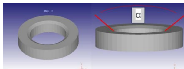
Fig 2. Bottom Die Geometry Variation
